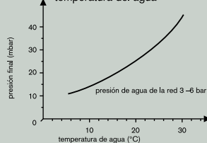
Presión final en función de la temperatura del agua
